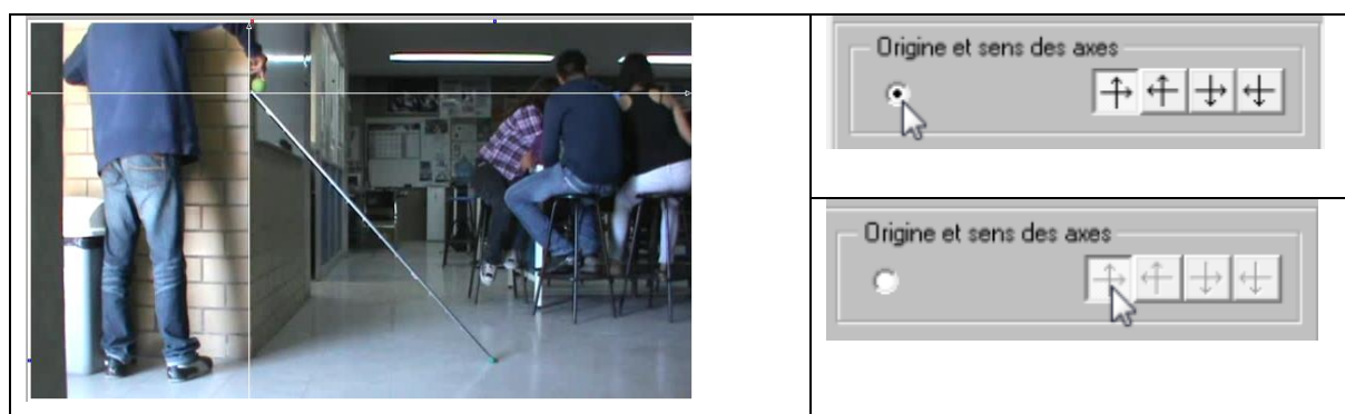
Figura 1: (Izquierda) Un estudiante deja caer una pelota por el plano inclinado. La captura de pantalla muestra los ejes cartesianos producido por el software AviMéca (derecha) y la configuración del sistema de referencia en el mismo (derecha).
